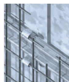
Sistema di aggancio senza saldature della rete al controtelaio (brevettato)
