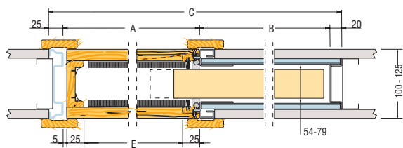
Dimensioni telaio intonaco in mm
