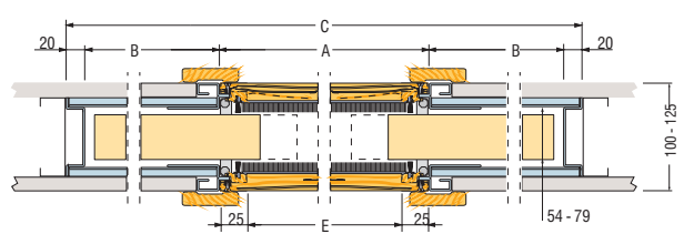
Dimensioni telaio intonaco in mm
