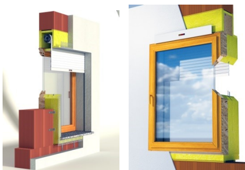
Le soluzioni RoverBlok (sinistra) e RoverBlok VMC (destra) di Roverplastik impiegate per la realizzazione della residenza in legno di Carpi (MO)
