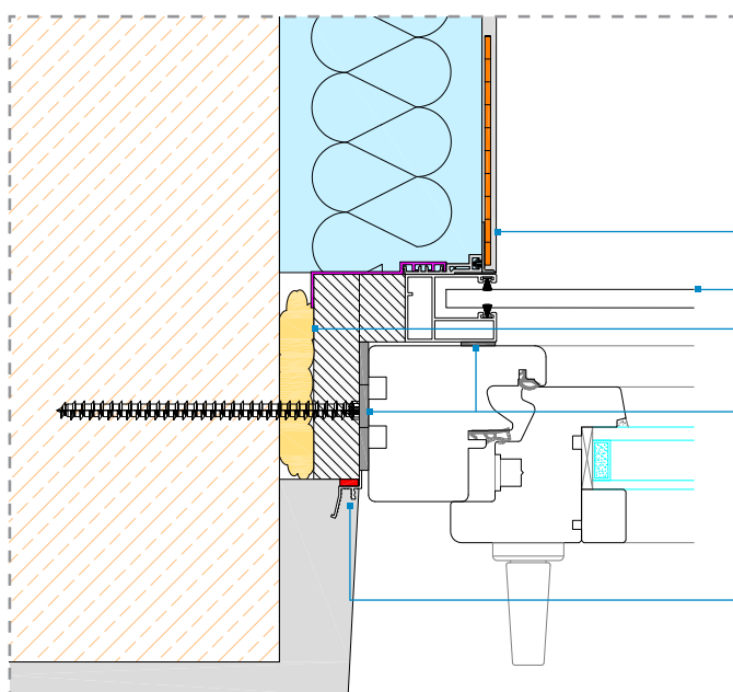
Particolari dei complementi di posa
